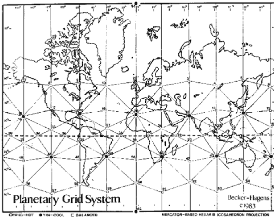
Becker-Hagens Grid
